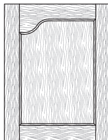
Style: 2202L PC: 202 Frame: PC102 x 0.6 Min. Size: 6½x7¼
