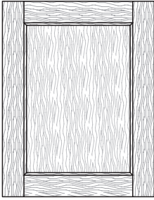
Style: 40 PC: 201 Frame: PC101 x 0.6 Min. Size: 6½x6
