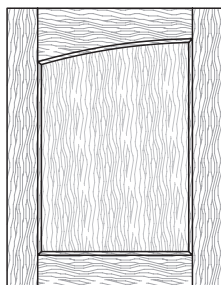
Style: 2002L PC: 202 Frame: PC102 x 0.6 Min. Size: 6½x7¼
