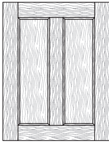
Style: 4040 PC: 203 Frame: PC103 x 0.6 Min. Size: 9¼x6½
