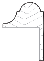
☐ #894-LF PC: M103 Sq Ft: .72 3/4"W 1 1/32"T
