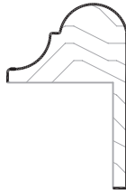
☐ #1264-LF PC: M103 Sq Ft: .72 1 1/16"W 1 1/32"T
