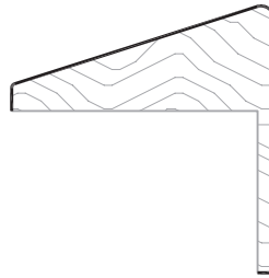
#3047-LF PC: M103 Sq Ft: .85 1 1/4"W 1 1/32"T
