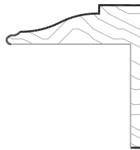
#3158-LF PC: M103 Sq Ft: .72 1"W 1 1/32"T
